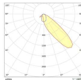
L5 Lens
