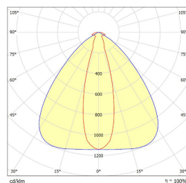
L9 Lens
